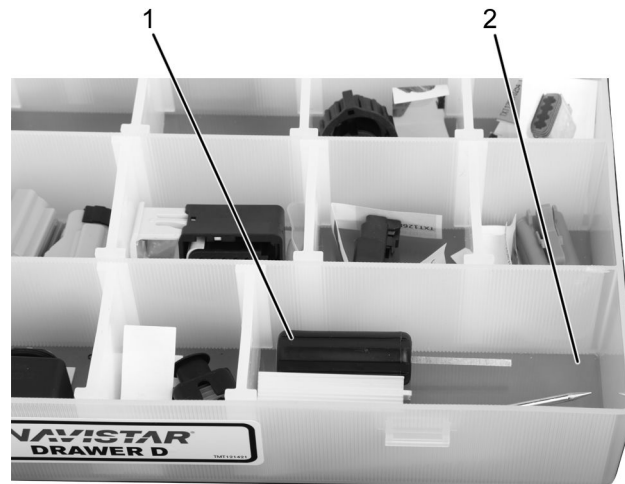
Figure 6. Emplacement de l'outil 49307 dans le tiroir D.
