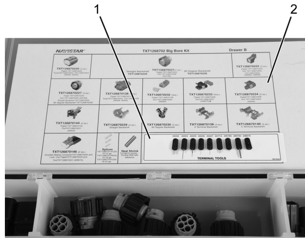
Figure 8. Autocollant de recouvrement du tiroir B.
