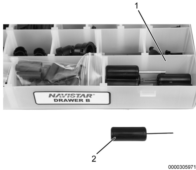
Figure 7. Emplacement de l'outil 49307 dans le tiroir B.
