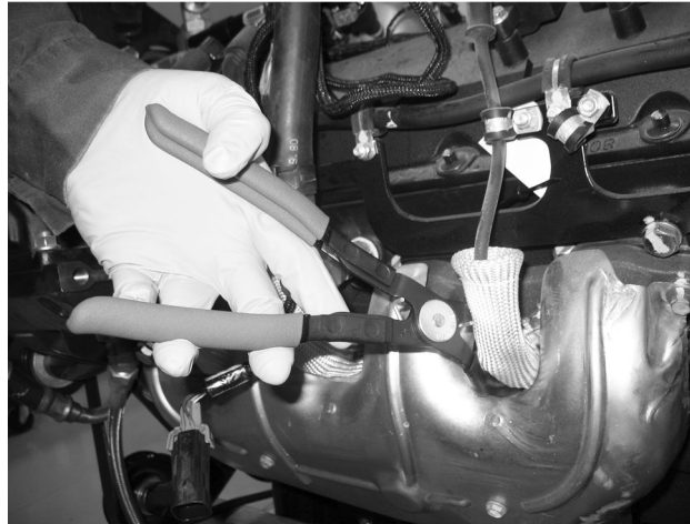
Figura 2. Pinza para funda de bujía.
