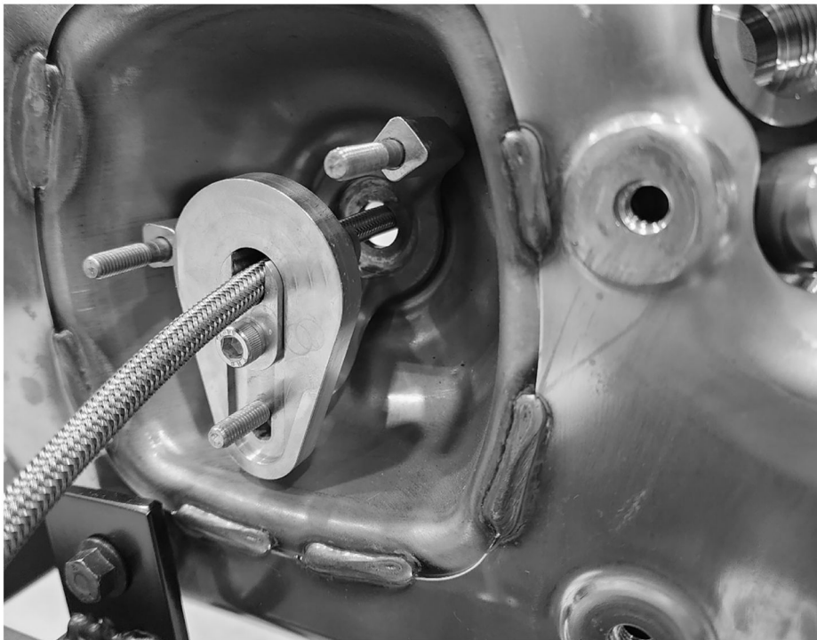
Figura 2. Kit de limpieza del depósito de DEF
