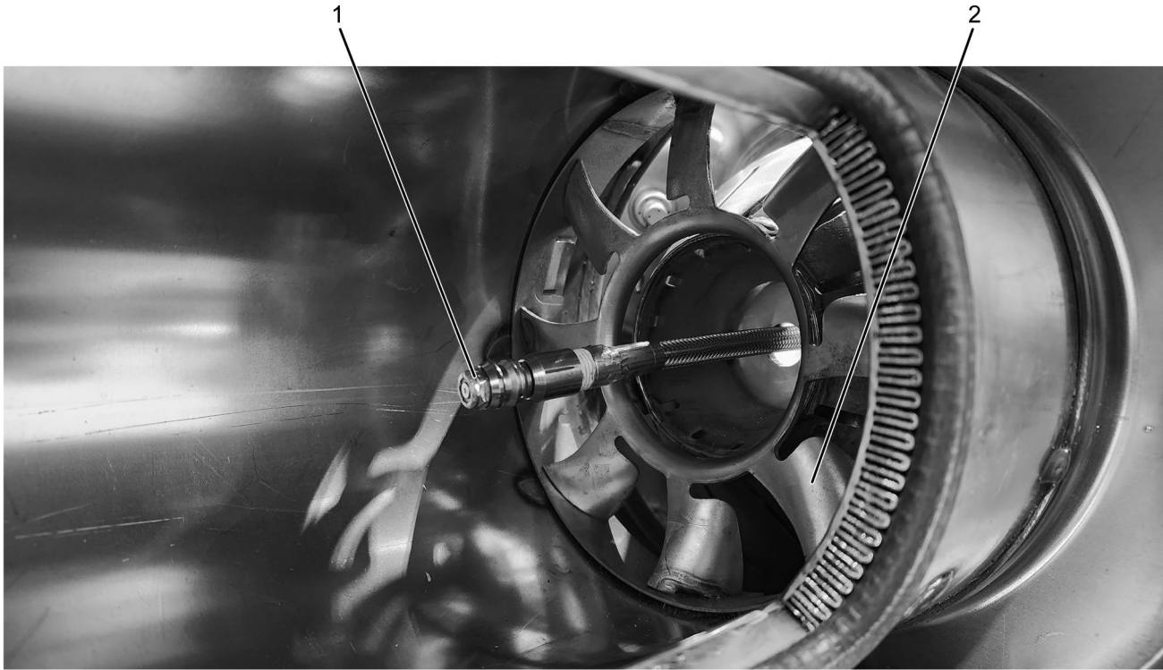
Figura 3. Kit de limpieza del depósito de DEF
